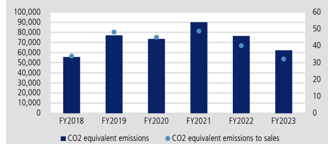
圖 14: 碳排量
